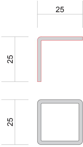
Standardprofile: Vierkant-, Winkelprofil
