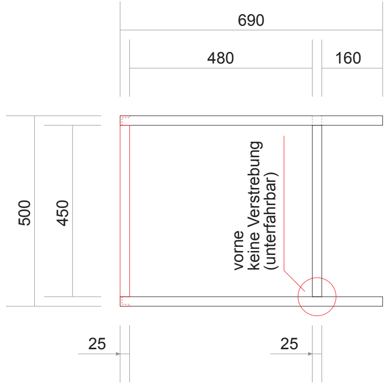
Ansicht Seite
