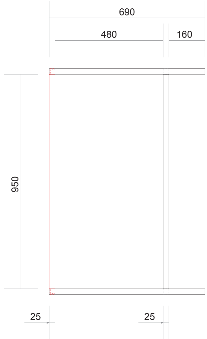
Ansicht frontal
